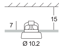
Ø 10,2 Ø 7,7 dimensione foro per incasso cut out hole dimension
