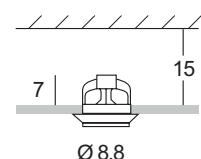
Ø 8,8 Ø 7,7 dimensione foro per incasso cut out hole dimension
