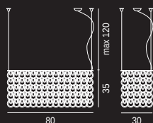
Minigiogali SP RET 2 3x100W E27 inc.
