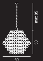
Minigiogali SP 60 3x100W E27 inc.
