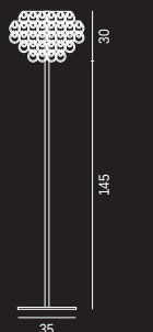
Minigiogali PT NV 3x100W E27 inc.
