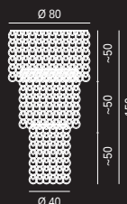
Minigiogali PL CAS 3 8x100W E27 inc.
